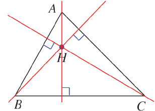
المثلث ABC حاد الزوايا
