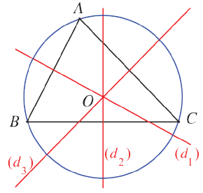
المثلث ABC حاد الزوايا
